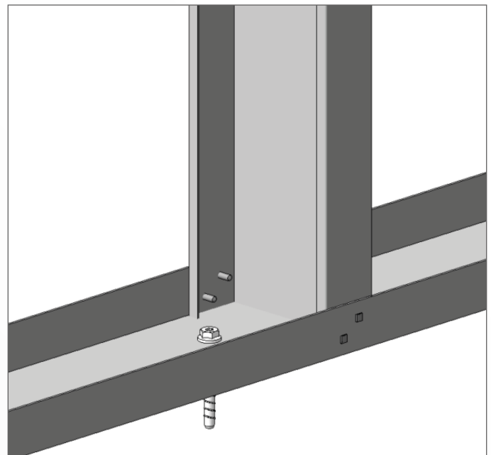
Abbildung 2: Detail Verschraubung C- mit U-Profilen
