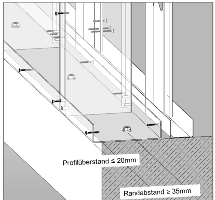
Abbildung 1: Bodenanschluss mit Profilüberstand
